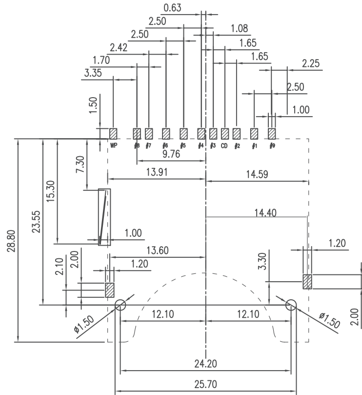
P.C.B LAYOUT
